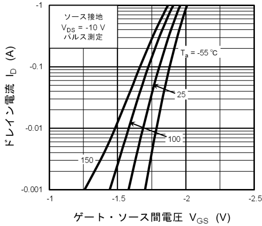
図 8.7 I_D - V_{GS}
