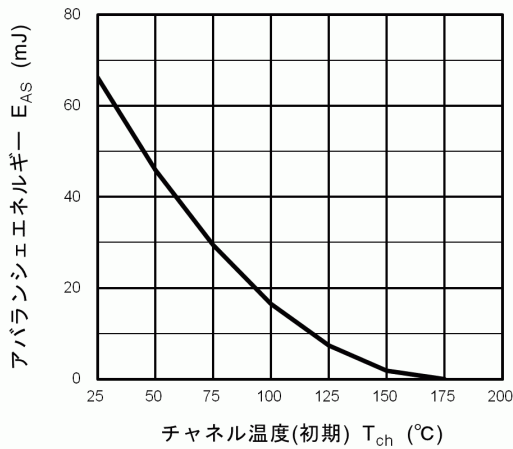
図 8.15 E_{AS} - T_{ch}
