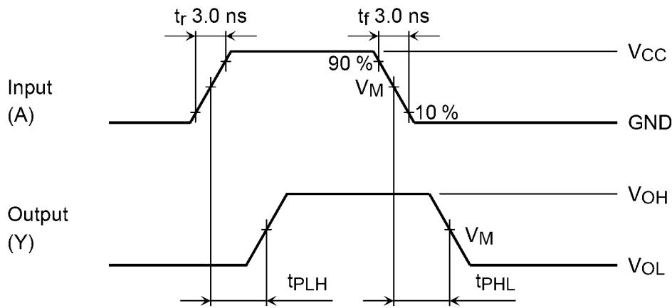
图 9.8.1 t_{PLH} , t_{PHL}
