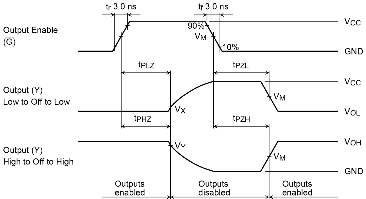
图 9.8.2 t_{PLZ} , t_{PHZ} , t_{PZL} , t_{PZH}
