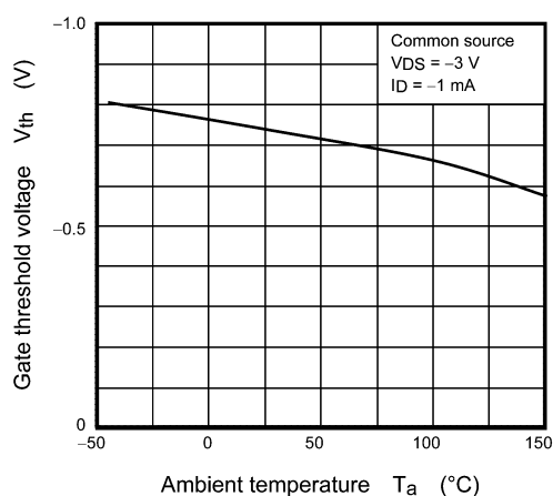
Fig. 9.6 V_{th} - T_a
