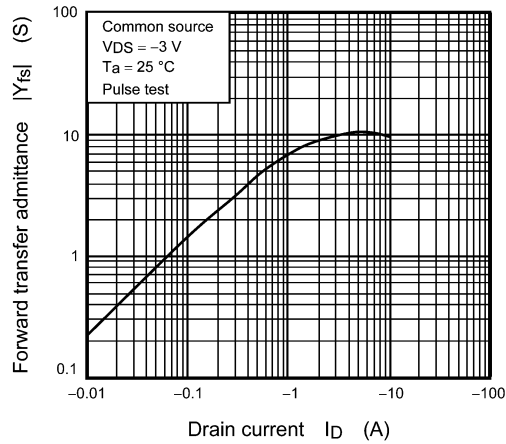
Fig. 9.7 |Y_{fs}| - I_D
