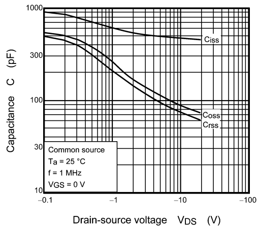
Fig. 9.9 C - V_{DS}
