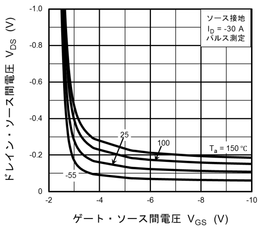
図 8.3 V_{DS} - V_{GS}
