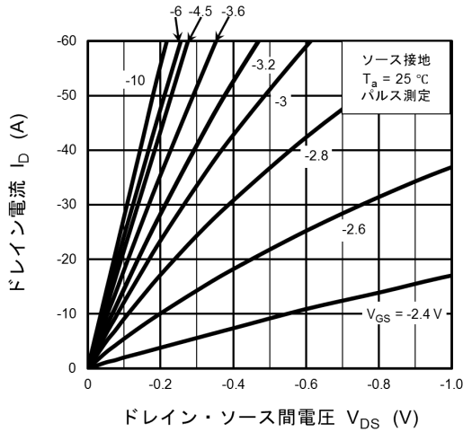
図 8.1 I_D - V_{DS}
