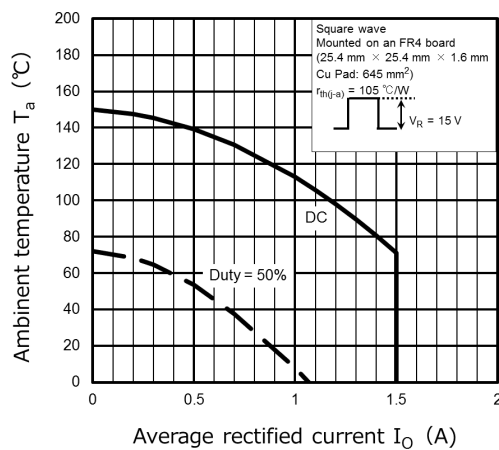
図 9.6 T_a - I_O
