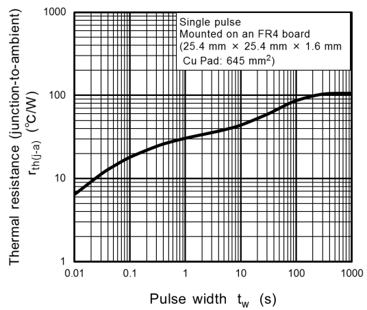
Fig. 9.4 r_{th} - t_w
