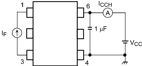
图 13.1.5 I CCH 测定回路
