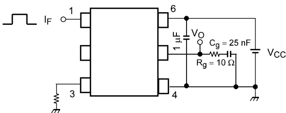
图 13.1.7 伝搬遅延時間測定回路, 波形
