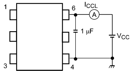
图 13.1.6 I CCL 测定回路
