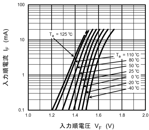
図 13.2.1 I_F - V_F
