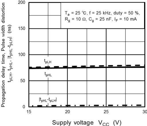
Fig. 13.2.13 t pLH , t pHL , |t pHL - t pLH | - V CC
