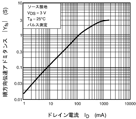
図 7.1.7 |Y_{fs}| - I_D
