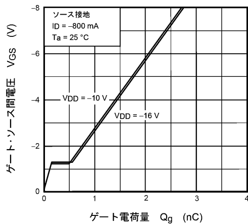
図 7.2.12 ダイナミック入力特性
