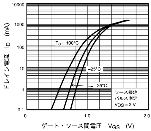
図 7.1.2 I_D - V_{GS}
