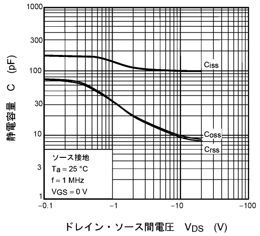
図 7.2.10 C - V_{DS}
