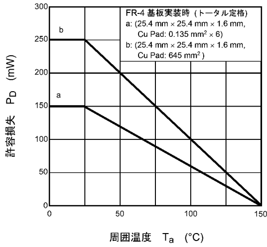
図 7.3.1 P_D - T_a
