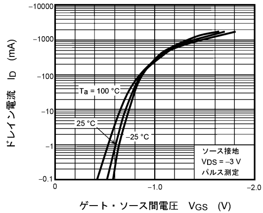
図 7.2.2 I_D - V_{GS}
