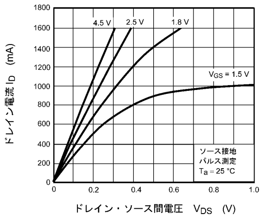
図 7.1.1 I_D - V_{DS}
