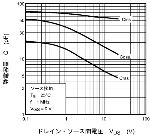
図 7.1.9 C - V_{DS}
