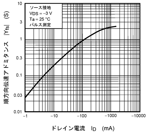
図 7.2.8 |Y_{fs}| - I_D
