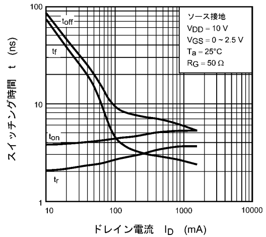
図 7.1.10 t - I_D
