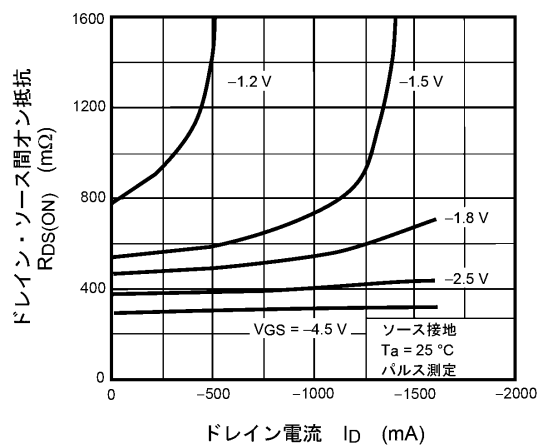
図 7.2.6 R_{DS(ON)} - I_D
