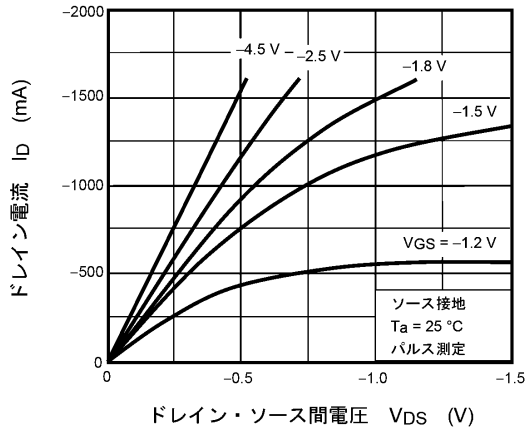
図 7.2.1 I_D - V_{DS}
