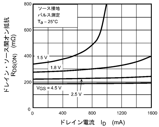
図 7.1.4 R_{DS(ON)} - I_D
