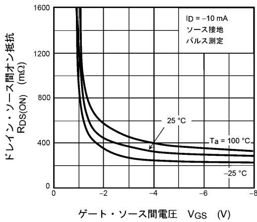
図 7.2.3 R_{DS(ON)} - V_{GS}
