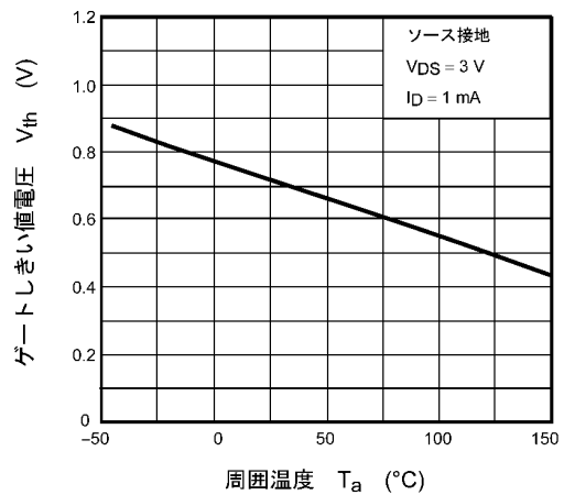
図 7.1.6 V_{th} - T_a
