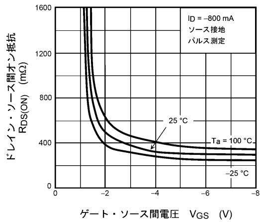
図 7.2.4 R_{DS(ON)} - V_{GS}
