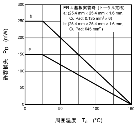
図 7.3.1 P_D - T_a
