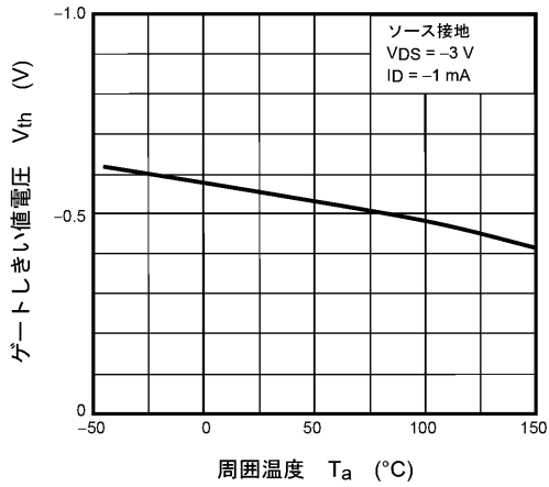
図 7.2.7 V_{th} - T_a
