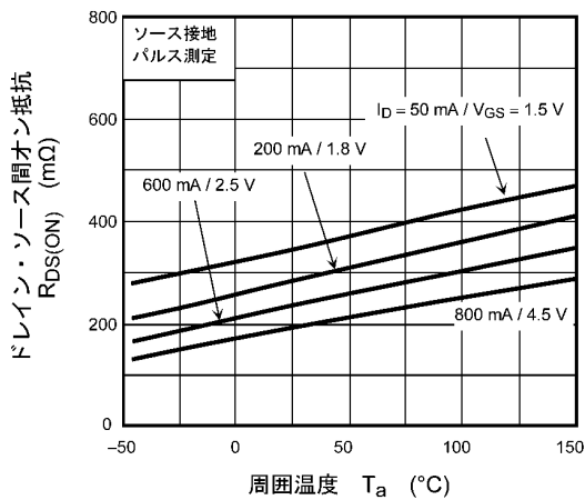
図 7.1.5 R_{DS(ON)} - T_a
