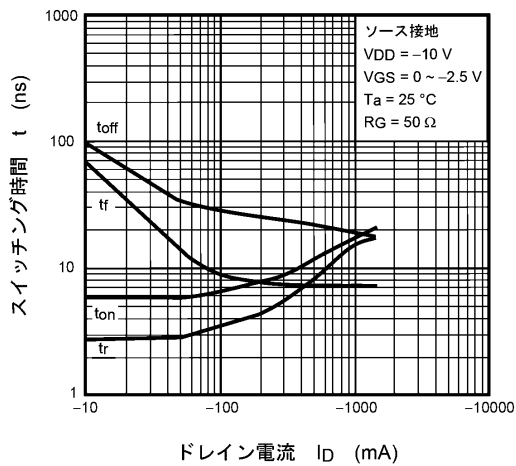
図 7.2.11 t - I_D
