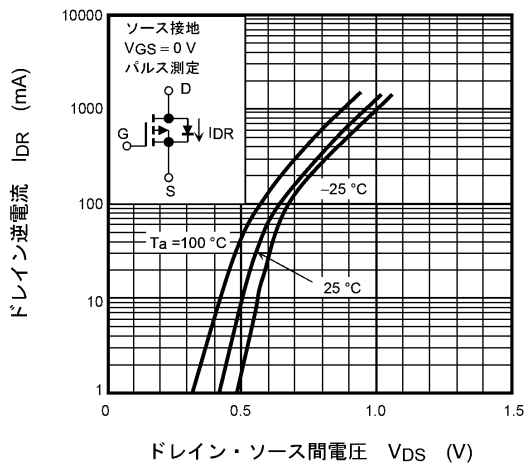
図 7.2.9 I_{DR} - V_{DS}
