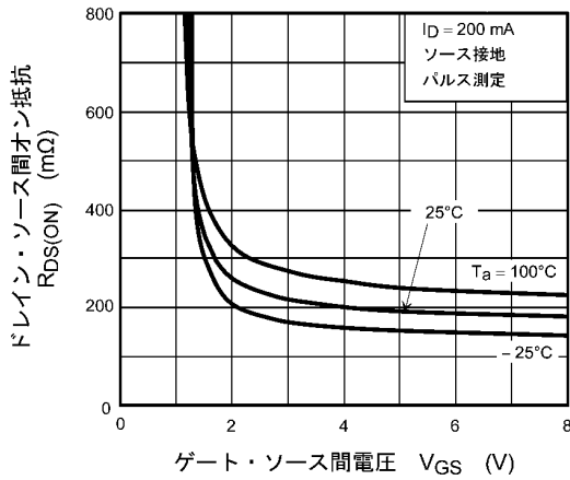
図 7.1.3 R_{DS(ON)} - V_{GS}
