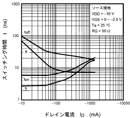
図 7.11 t - I_D
