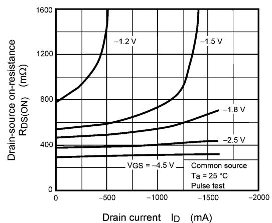
Fig. 7.6 R_{DS(ON)} - I_D
