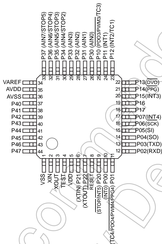
図 1-1 ピン配置図
