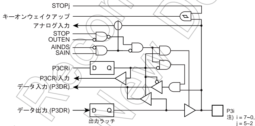
図 5-5 P3 ポート
