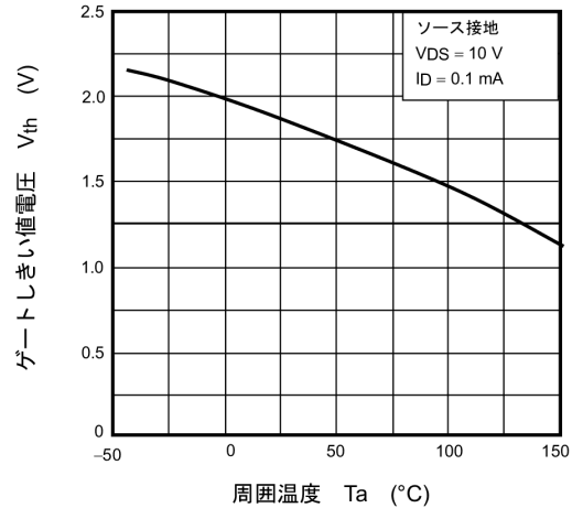
図 8.6 V_{th} - T_a
