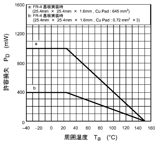
図 8.12 P_D - T_a
