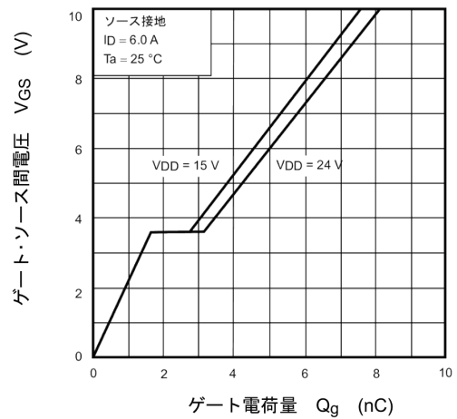
図 8.10 ダイナミック入力特性
