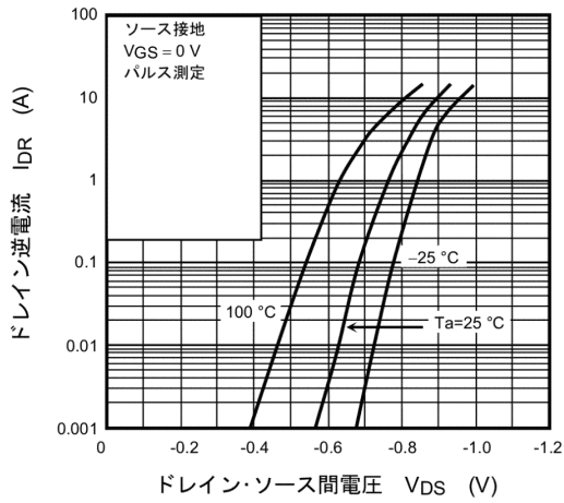
図 8.7 I_{DR} - V_{DS}
