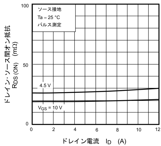
図 8.4 R_{DS(ON)} - I_D
