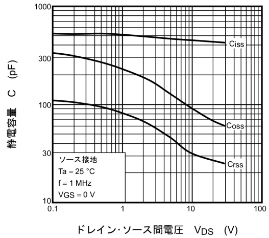
図 7.8 C - V_{DS}
