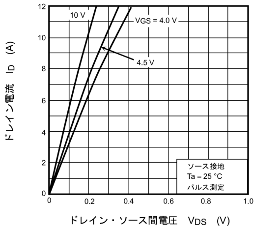
図 7.1 I_D - V_{DS}
