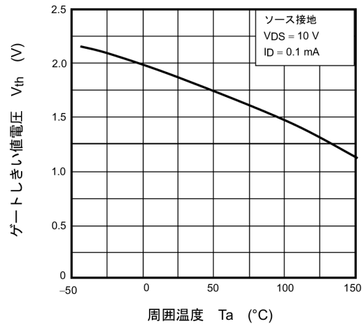
図 7.6 V_{th} - T_a
