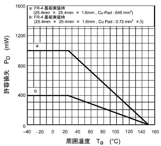
図 7.12 P_D - T_a
