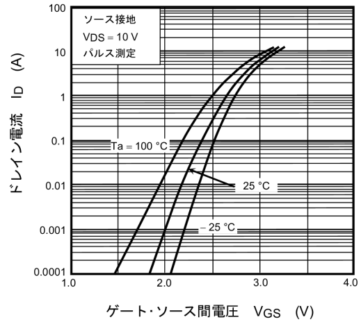
図 8.2 I_D - V_{GS}
