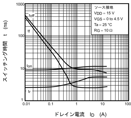
図 7.9 t - I_D
