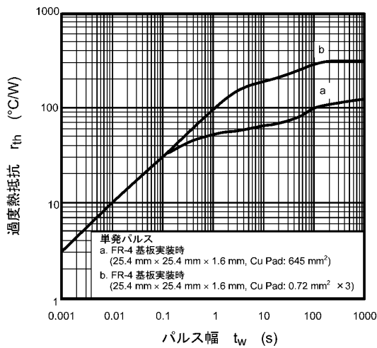
図 7.11 r_{th} - t_w
