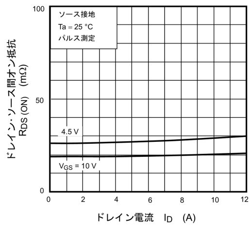
図 7.4 R_{DS(ON)} - I_D
