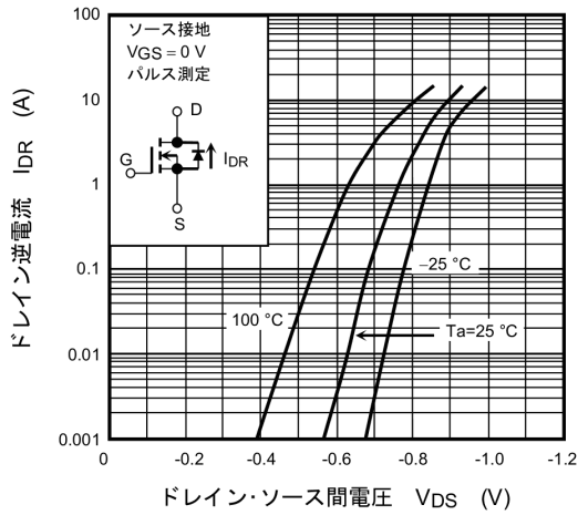
図 7.7 I_{DR} - V_{DS}
