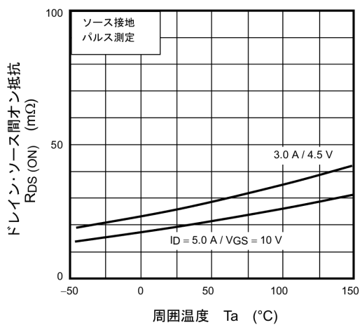
図 7.5 R_{DS(ON)} - T_a
