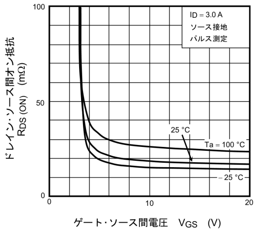
図 7.3 R_{DS(ON)} - V_{GS}
