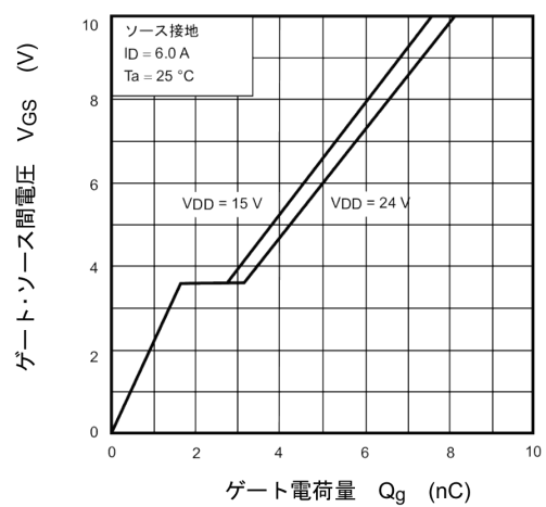
図 7.10 ダイナミック入力特性
