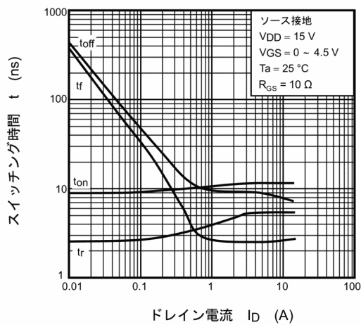
図 8.9 t - I_D
