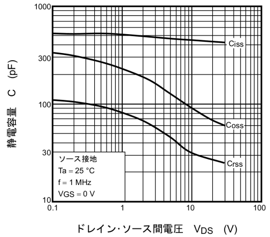
図 8.8 C - V_{DS}
