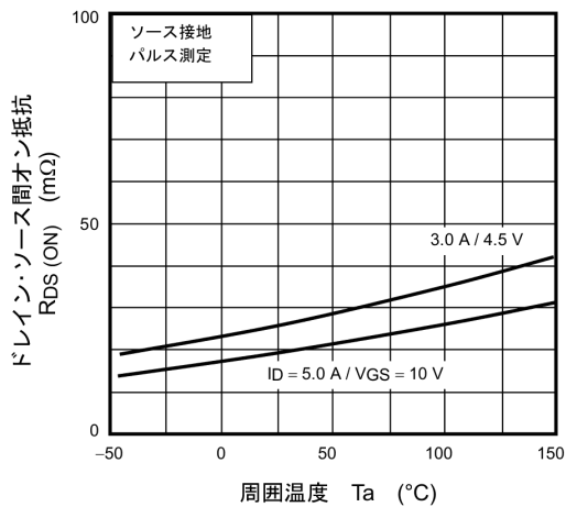
図 8.5 R_{DS(ON)} - T_a
