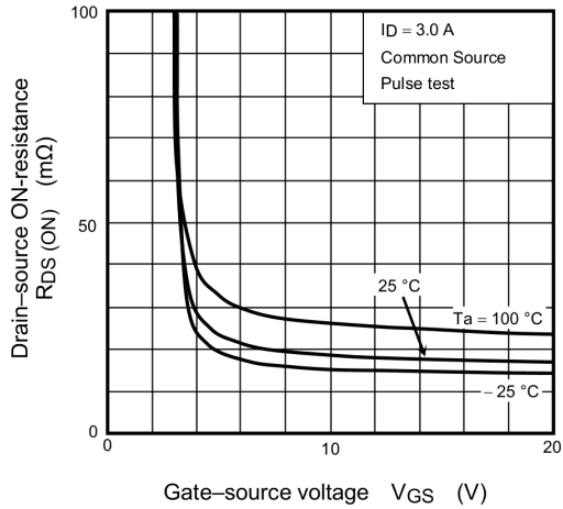
Fig. 8.3 R_{DS(ON)} - V_{GS}
