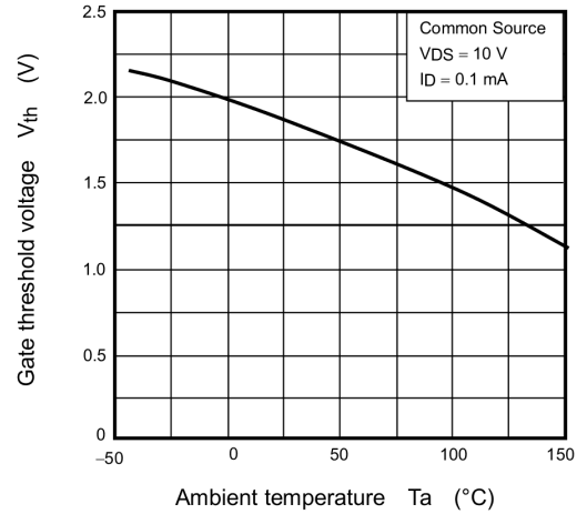
Fig. 8.6 V_{th} - T_a
