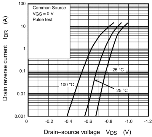
Fig. 8.7 I_{DR} - V_{DS}
