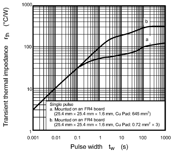
Fig. 8.11 r_{th} - t_w
