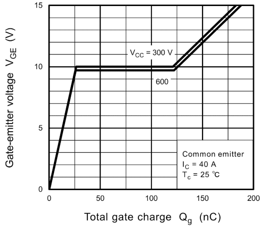
Fig. 8.7 V_{GE} - Q_g
