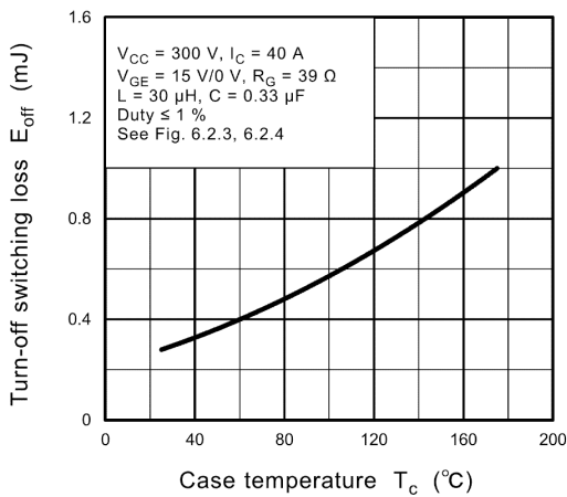
Fig. 8.17 E_{off} - T_c
