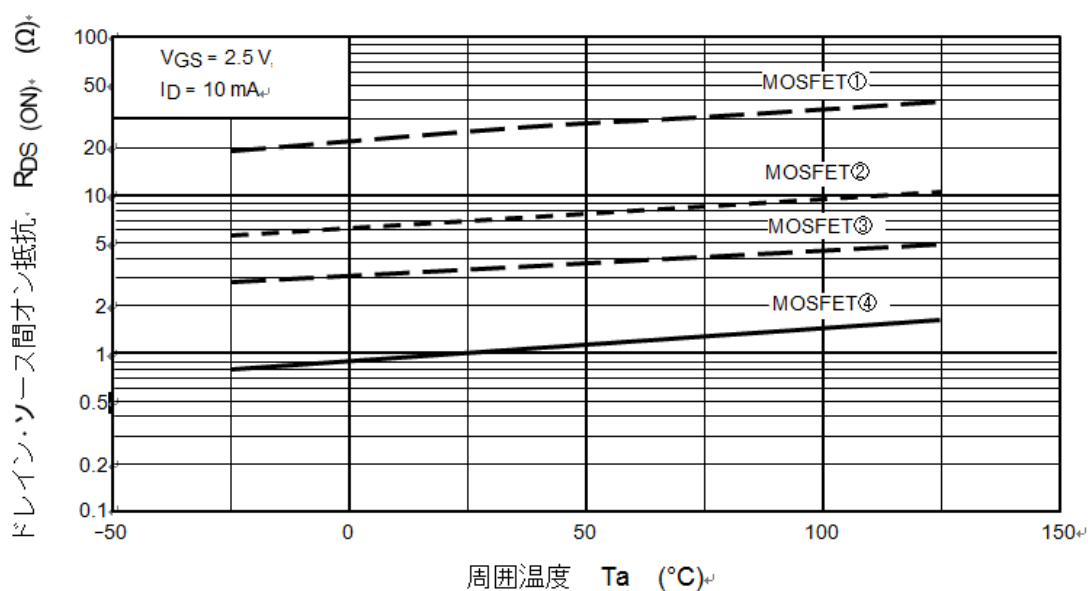
図 5.2 R_{DS(ON)} - T_a
