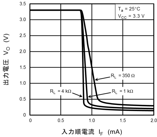
図 12.2.7 V_O - I_F
