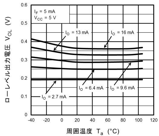
図 12.2.6 V_{OL} - T_a
