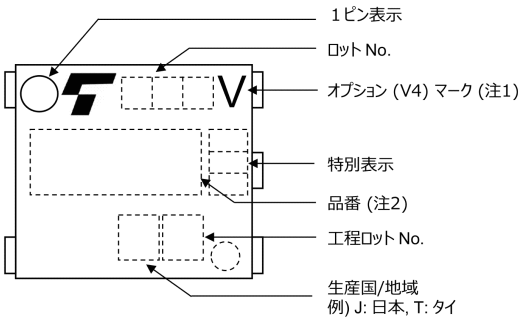
図 16.4 現品表示例
