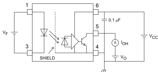
図 12.1.1 I_{OH} 測定回路
