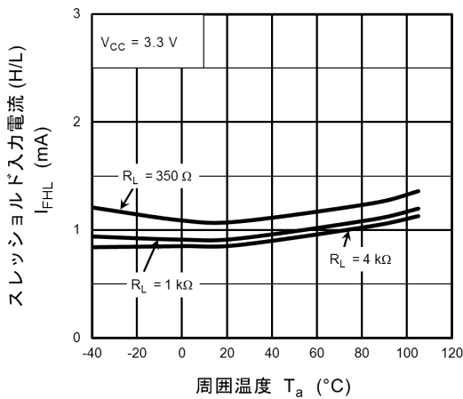
図 12.2.9 I_{FHL} - T_a
