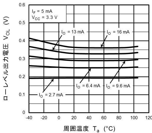
図 12.2.5 V_{OL} - T_a
