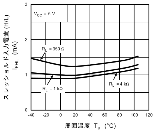
図 12.2.10 I_{FHL} - T_a
