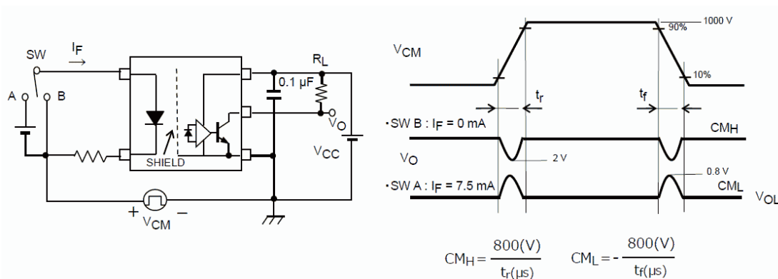
図 12.1.6 コモンモード過渡耐性測定回路, 波形
