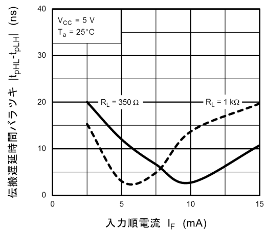
図 12.2.24 |t_{pHL} - t_{pLH}| - I_F
