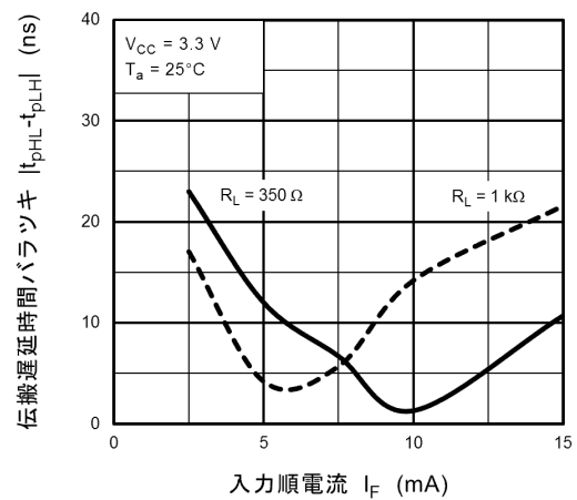
図 12.2.22 |t_{pHL} - t_{pLH}| - I_F
