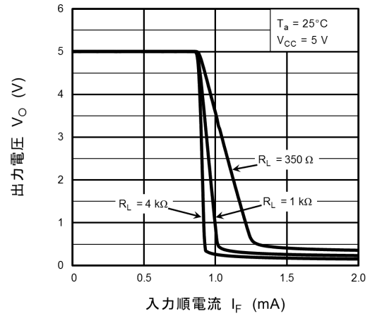
図 12.2.8 V_O - I_F
