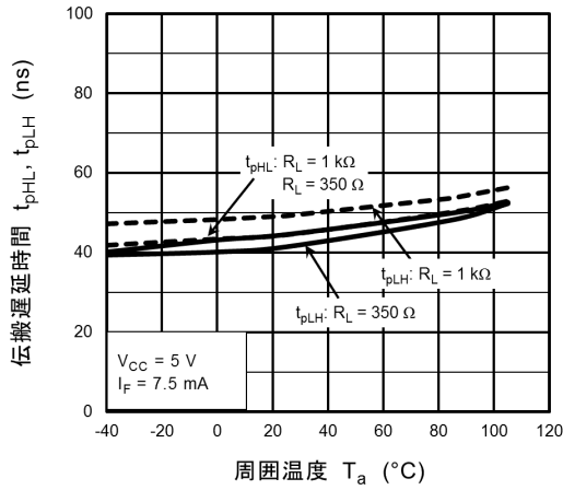
図 12.2.19 t_{pHL}, t_{pLH} - T_a
