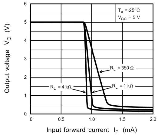
Fig. 12.2.8 V_O - I_F
