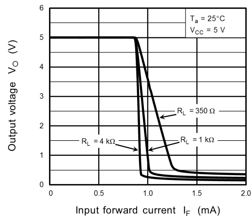
Fig. 12.2.8 V_O - I_F
