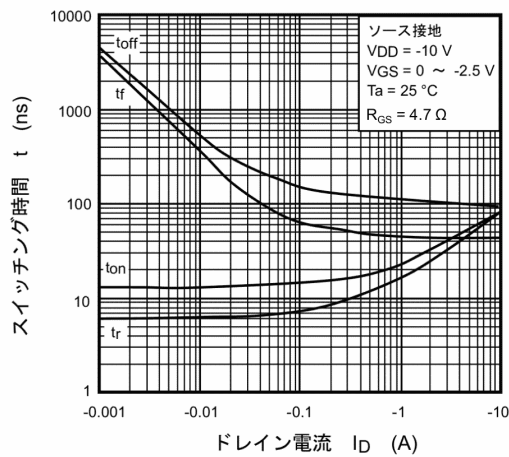
図 9.11 t - I_D
