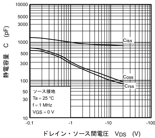
図 9.9 C - V_{DS}
