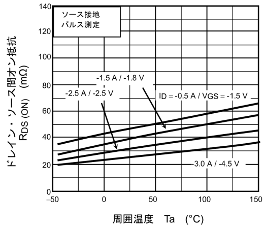
図 9.6 R_{DS(ON)} - T_a
