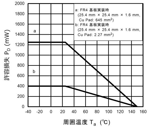
図 9.14 P_D - T_a
