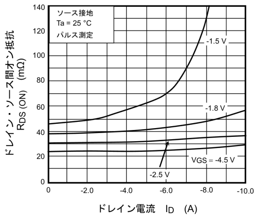
図 9.5 R_{DS(ON)} - I_D
