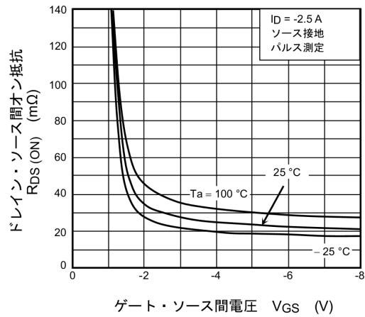
図 9.4 R_{DS(ON)} - V_{GS}
