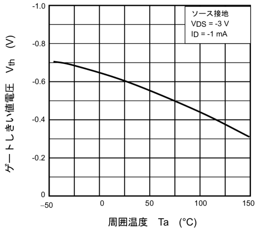
図 9.7 V_{th} - T_a
