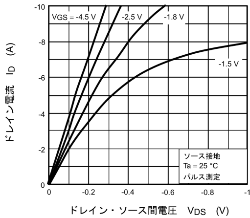
図 9.1 I_D - V_{DS}
