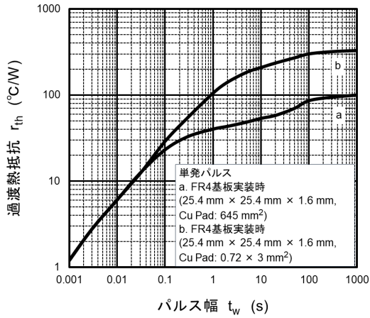
図 9.13 r_{th} - t_w
