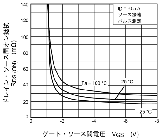
図 9.3 R_{DS(ON)} - V_{GS}
