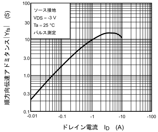
図 9.8 |Y_{fs}| - I_D
