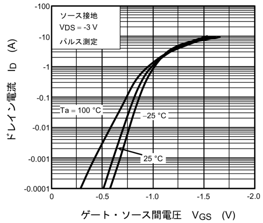
図 9.2 I_D - V_{GS}
