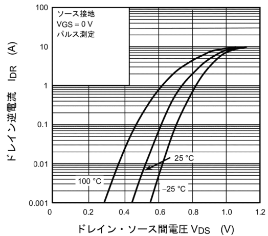
図 9.12 I_{DR} - V_{DS}
