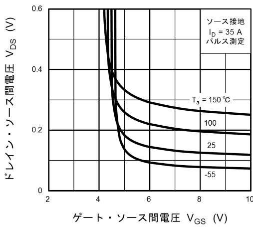
図 8.3 V_{DS} - V_{GS}
