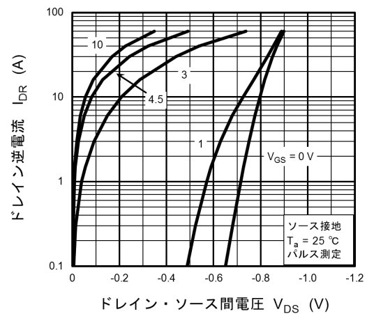
図 8.10 I_{DR} - V_{DS}
