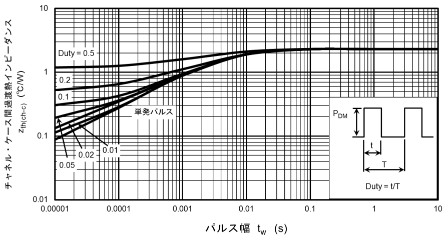
図 8.15 Z_{th(ch-c)} - t_w (最大値 (保証値))
