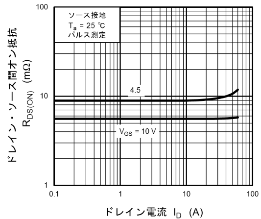
図 8.8 R_{DS(ON)} - I_D
