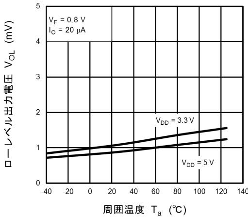
図 12.2.3 V_{OL} - T_a
