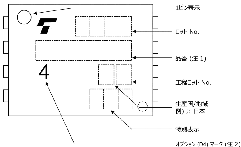
図 16.4 現品表示例
