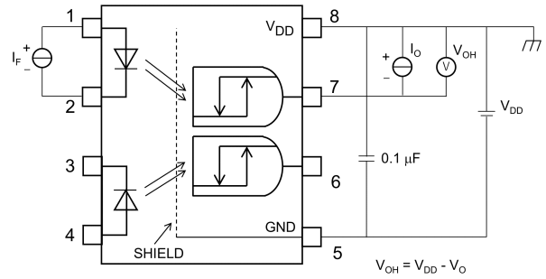
図 12.1.2 V_{OH} 測定回路
