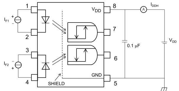
図 12.1.4 I_{DDH} 測定回路
