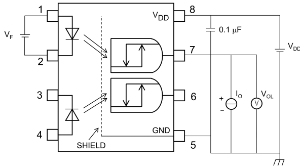
図 12.1.1 V_{OL} 測定回路
