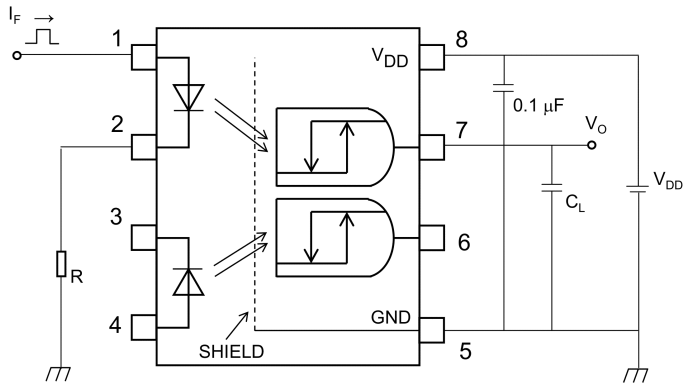
図 12.1.6 伝搬遅延時間測定回路, 波形
