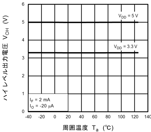
図 12.2.5 V_{OH} - T_a
