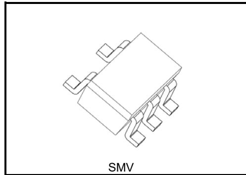
質量: SMV (SOT-25)(SC-74A) : 16 mg (標準)
