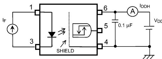
図 12.1.4 IDD_H測定回路
