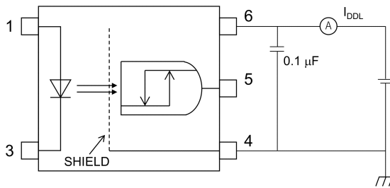
図 12.1.3 I_{DDL} 測定回路
