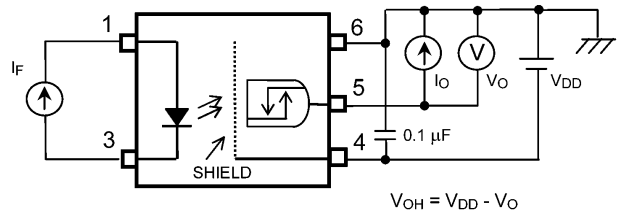
図 12.1.2 VOH測定回路
