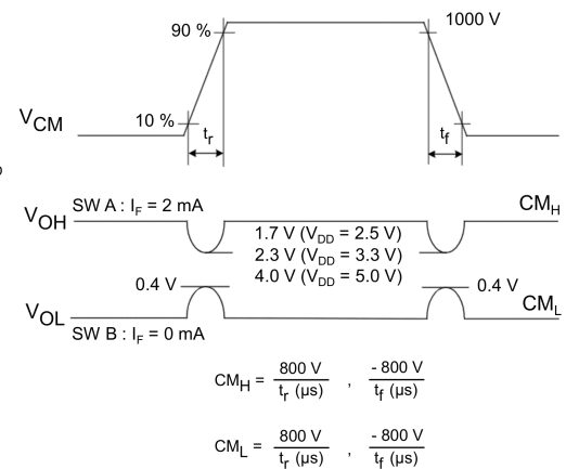
図 12.1.6 コモンモード過渡耐性測定回路, 波形
