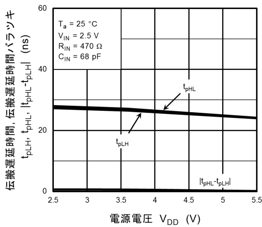
図 12.2.14 t_{pHL} , t_{pLH} , |t_{pHL} - t_{pLH}| - V_{DD}
