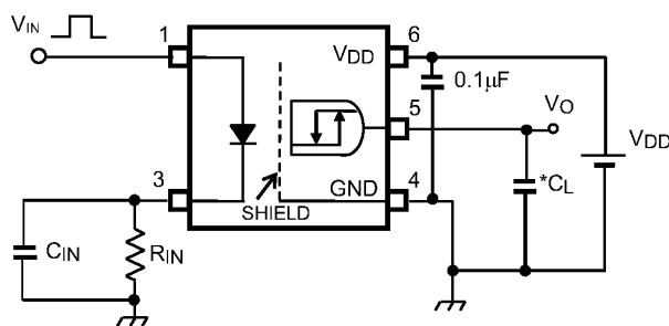
図 12.1.5 伝搬遅延時間測定回路, 波形
