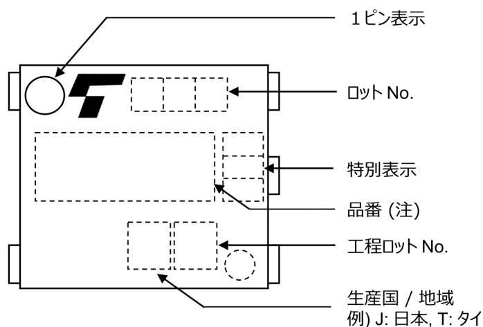
図 16.3 現品表示例 (注)
