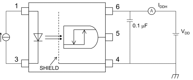
図 12.1.4 I_{DDH} 測定回路
