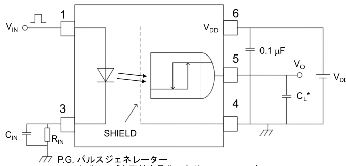
図 12.1.5 伝搬遅延時間測定回路, 波形
