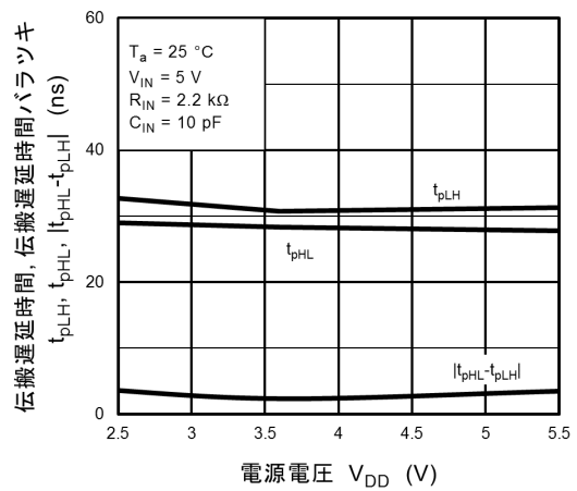
図 12.2.15 t_{pHL} , t_{pLH} , |t_{pHL} - t_{pLH}| - V_{DD}
