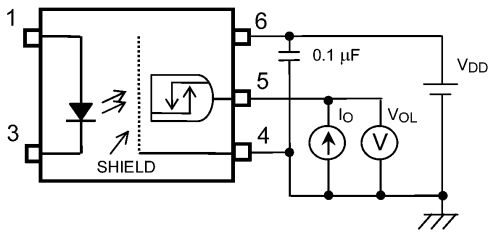
図 12.1.1 VOL測定回路
