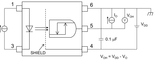
図 12.1.2 V_{OH} 測定回路
