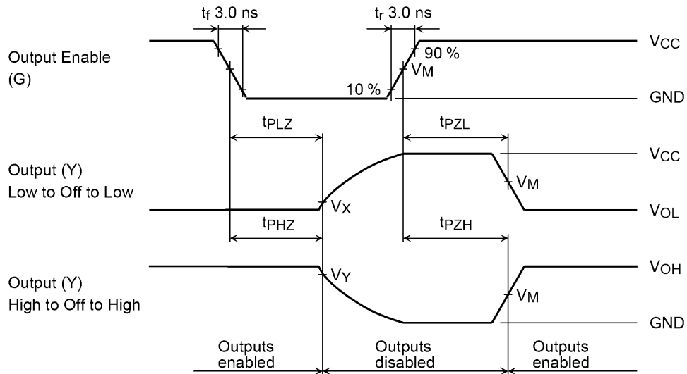
图 9.6.2 t PLZ , t PHZ , t PZL , t PZH
