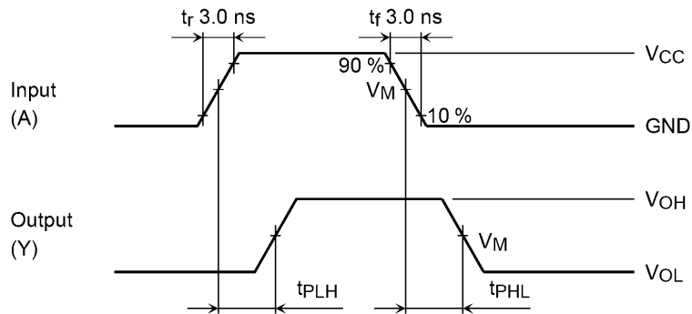
图 9.6.1 t PLH , t PHL
