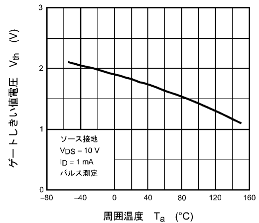
図 8.8 V_{th} - T_a
