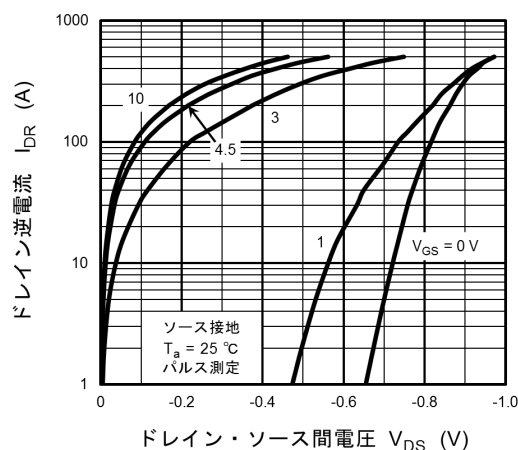
図 8.6 I_{DR} - V_{DS}
