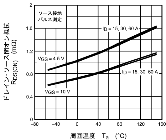
図 8.9 R_{DS(ON)} - T_a
