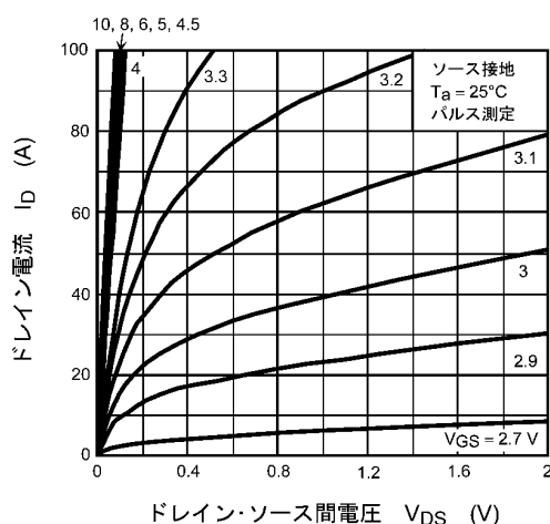
図 8.2 I_D - V_{DS}
