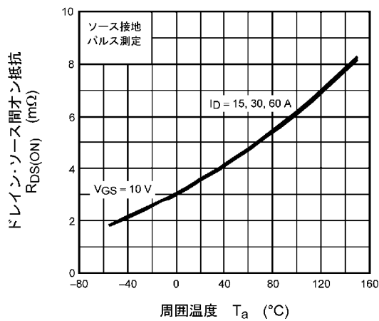
図 8.9 R_{DS(ON)} - T_a
