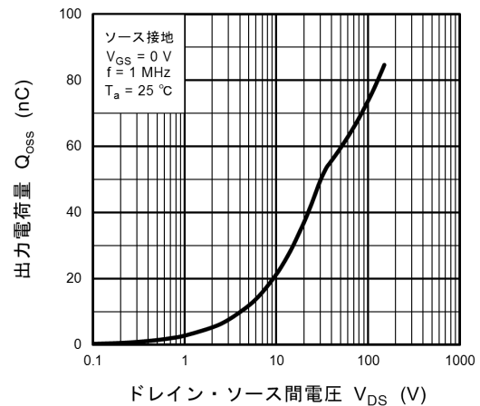
図 8.12 Q_{oss} - V_{DS}
