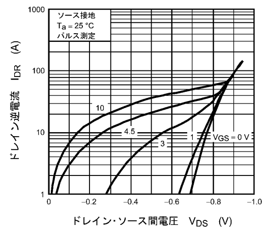
図 8.6 I_{DR} - V_{DS}
