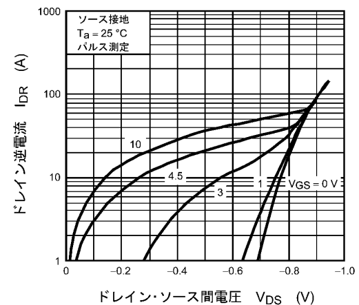
図 8.6 I_{DR} - V_{DS}
