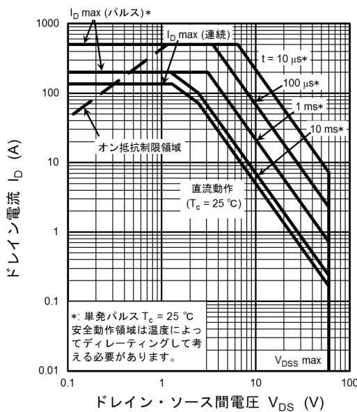
図 8.16 安全動作領域 (最大値 (保証値))
