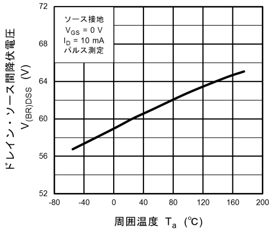
図 8.7 V_{(BR)DSS} - T_a
