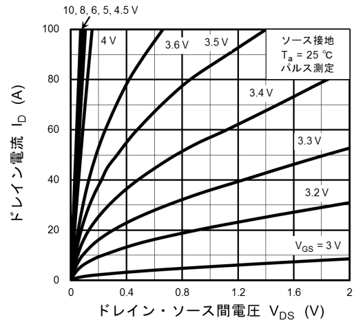
図 8.2 I_D - V_{DS}
