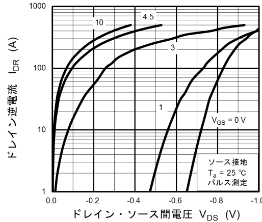
図 8.6 I_{DR} - V_{DS}
