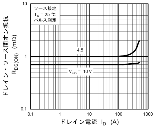
図 8.5 R_{DS(ON)} - I_D
