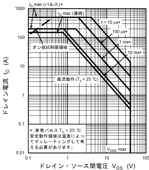
ドレイン・ソース間電圧 V_{DS} (V) 図 8.16 安全動作領域 (最大値 (保証値))
