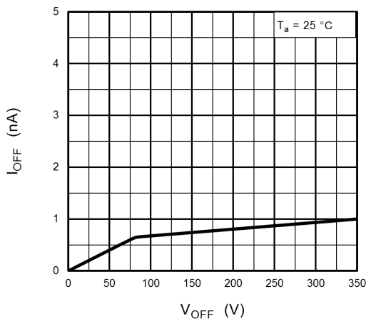
図 12.1.9 I_{OFF} - V_{OFF}
