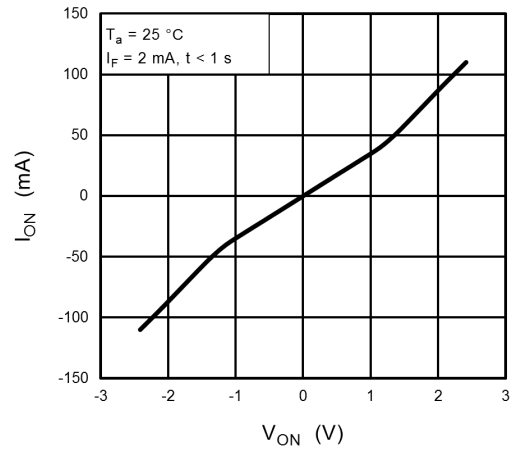
図 12.1.4 I_{ON} - V_{ON}
