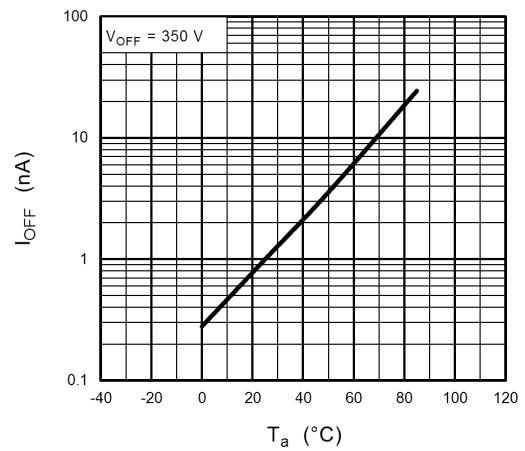
図 12.1.10 I_{OFF} - T_a
