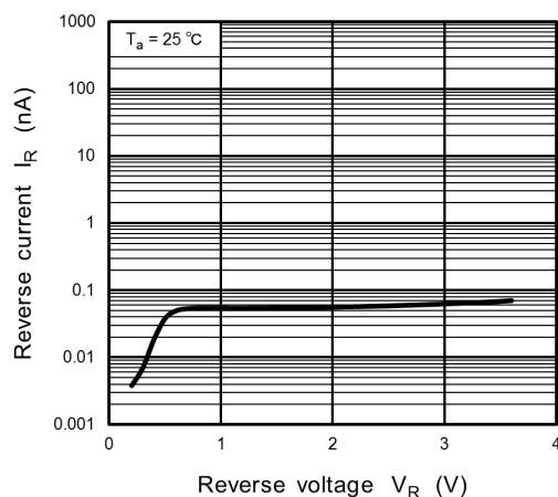
図 9.2 I_R - V_R
