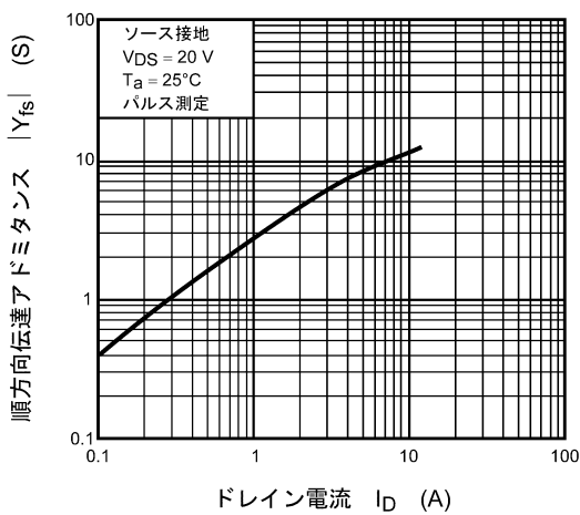
図 8.5 |Y_{fs}| - I_D
