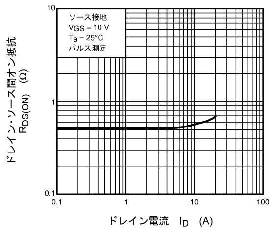
図 8.6 R_{DS(ON)} - I_D
