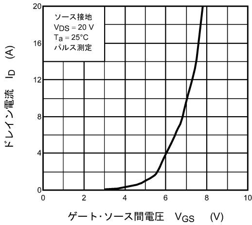
図 8.3 I_D - V_{GS}
