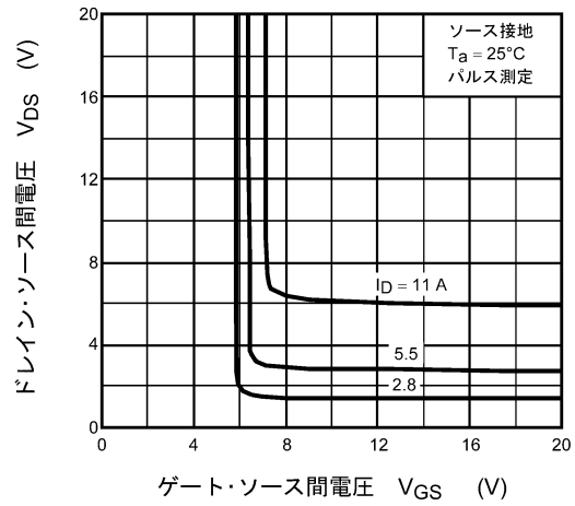
図 8.4 V_{DS} - V_{GS}
