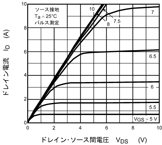
図 8.1 I_D - V_{DS}
