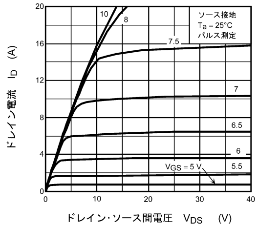
図 8.2 I_D - V_{DS}
