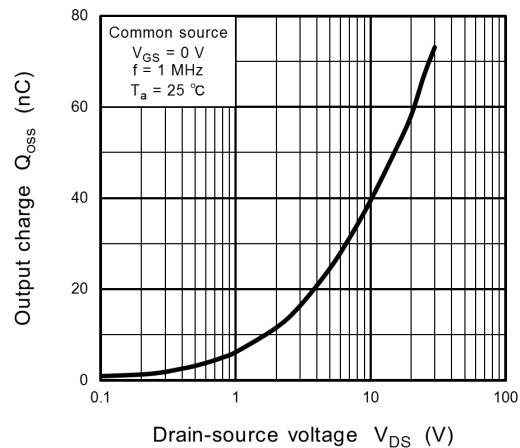
Fig. 8.12 Q_{oss} - V_{DS}
