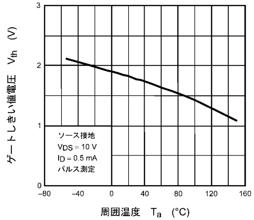
図 8.8 V_{th} - T_a
