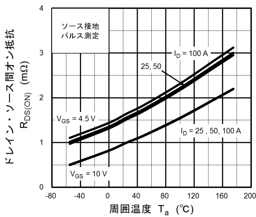
図 8.9 R_{DS(ON)} - T_a
