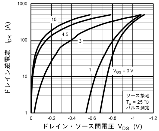
図 8.6 I_{DR} - V_{DS}
