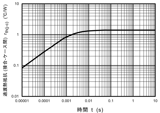
図 8.6 r_{th(j-c)} - t (最大値 (保証値)) (Per Leg)
