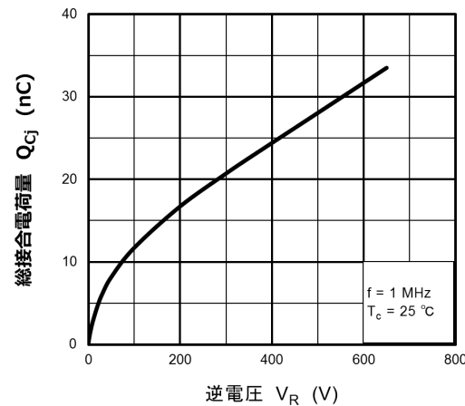
図 8.5 Q_{gj} - V_R
