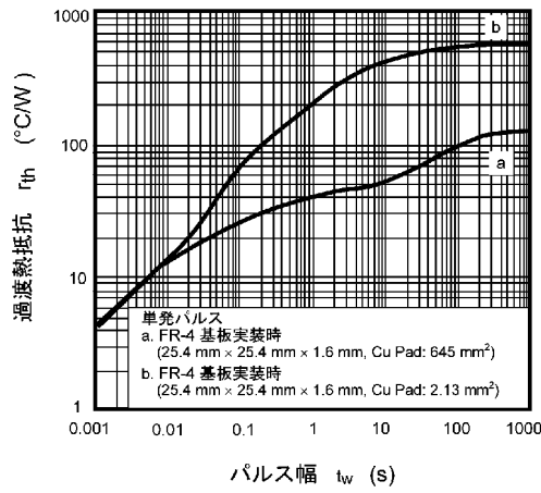
図 8.13 r_{th} - t_w
