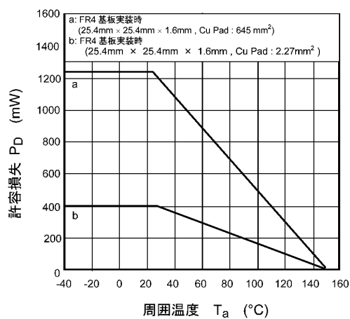
図 9.15 P_D - T_a
