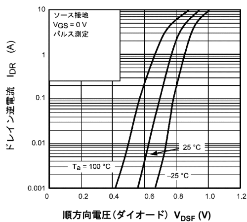
図 9.9 I_{DR} - V_{DSF}
