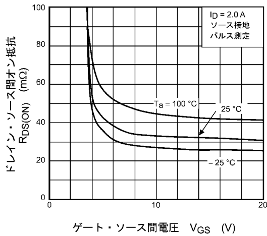
図 9.3 R_{DS(ON)} - V_{GS}
