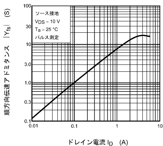
図 9.8 |Y_{fs}| - I_D
