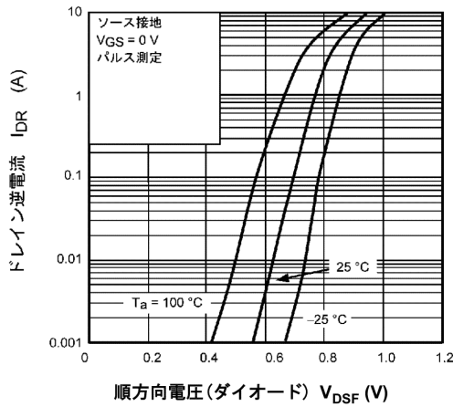
図 9.9 I_{DR} - V_{DSF}
