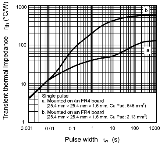
図 8.13 r_{th} - t_w
