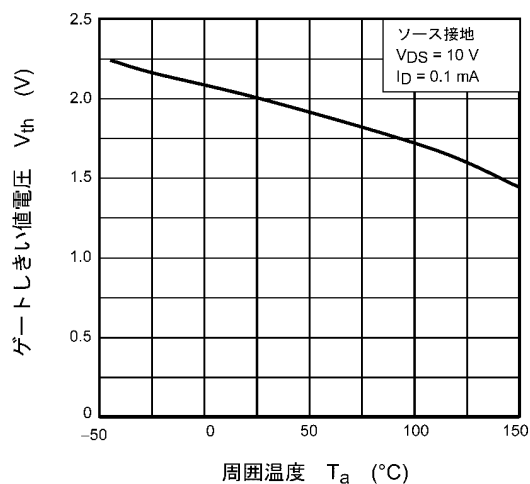
図 9.7 V_{th} - T_a
