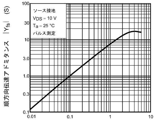
図 8.8 |Y_{fs}| - I_D
