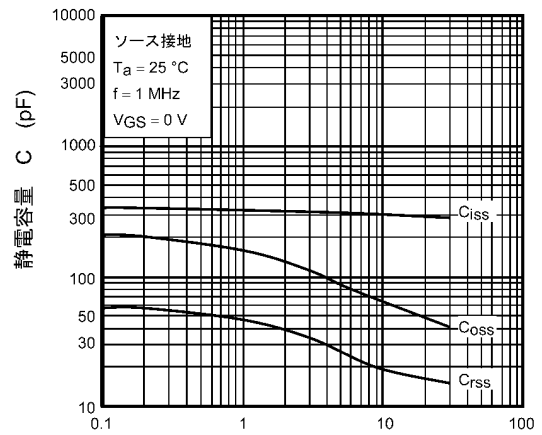
図 9.10 C - V_{DS}
