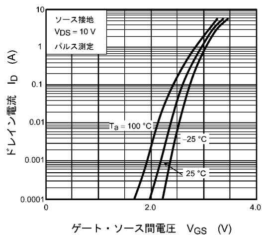
図 9.2 I_D - V_{GS}
