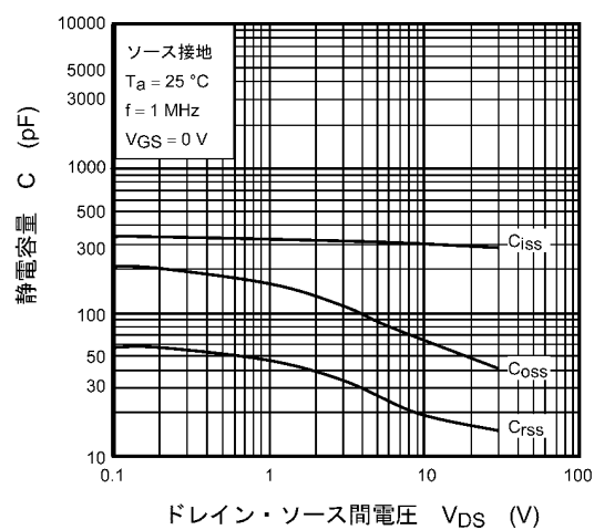
図 9.10 C - V_{DS}
