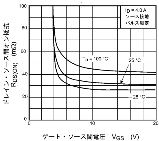
図 9.4 R_{DS(ON)} - V_{GS}
