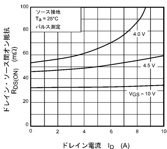
図 9.5 R_{DS(ON)} - I_D
