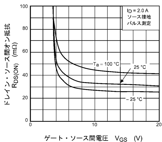
図 9.3 R_{DS(ON)} - V_{GS}
