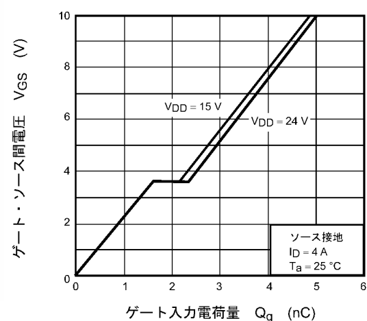
図 9.12 ダイナミック入力特性
