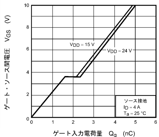
図 9.12 ダイナミック入力特性
