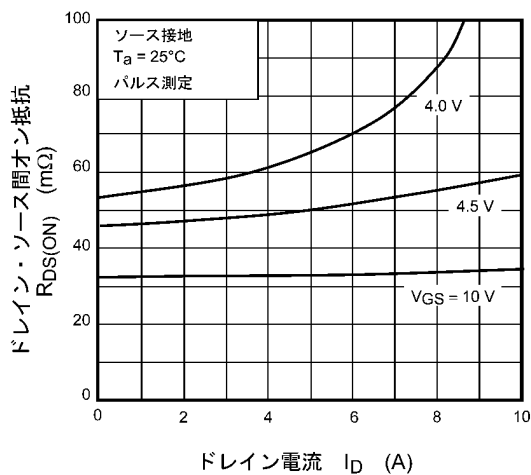
図 8.5 R_{DS(ON)} - I_D
