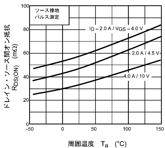
図 9.6 R_{DS(ON)} - T_a
