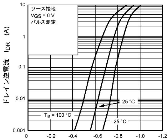
図 8.9 I_{DR} - V_{DS}
