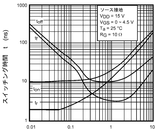
図 8.11 t - I_D
