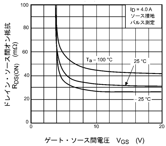
図 8.4 R_{DS(ON)} - V_{GS}
