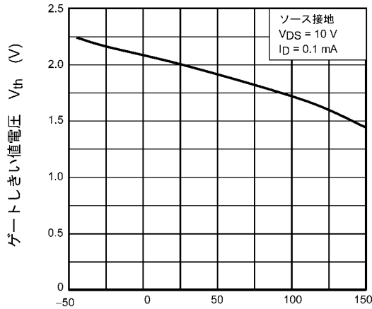
図 9.7 V_{th} - T_a
