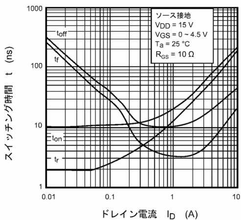
図 9.11 t - I_D
