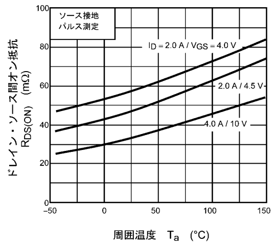
図 8.6 R_{DS(ON)} - T_a
