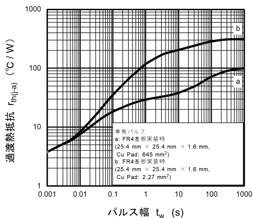
図 9.13 r_{th(j-a)} - t_w
