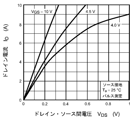
図 9.1 I_D - V_{DS}
