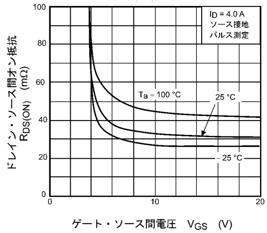
図 9.4 R_{DS(ON)} - V_{GS}
