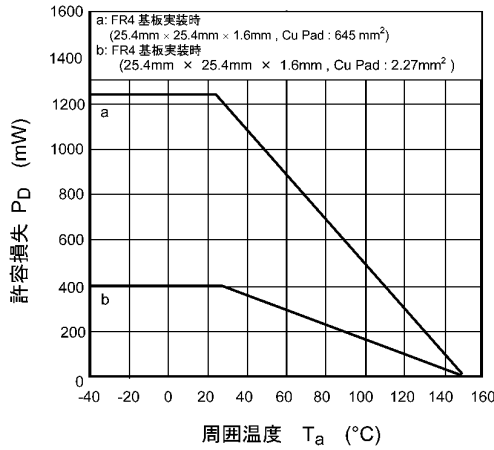
図 8.15 P_D - T_a
