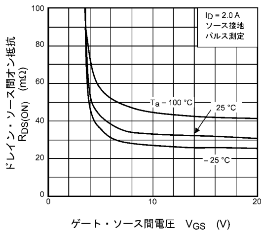
図 8.3 R_{DS(ON)} - V_{GS}
