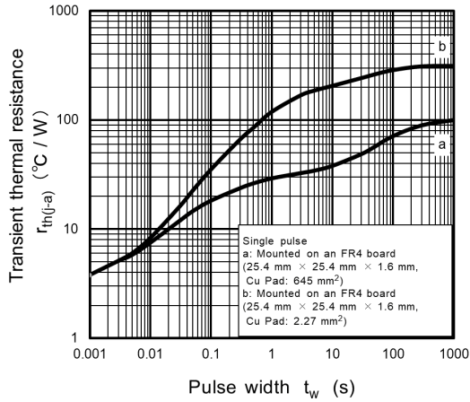
Fig. 9.13 r_{th(j-a)} - t_w
