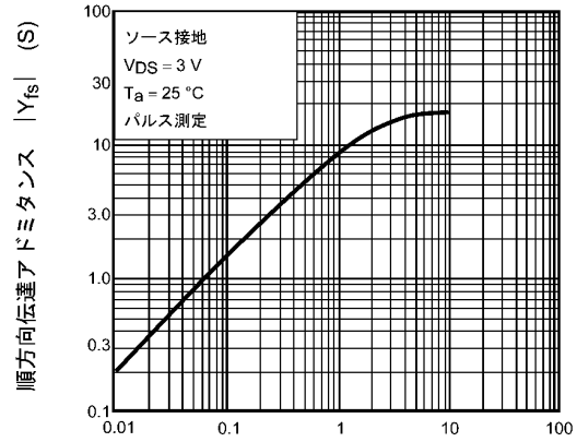
図 8.8 |Y_{fs}| - I_D
