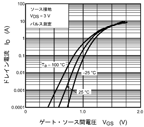
図 8.2 I_D - V_{GS}
