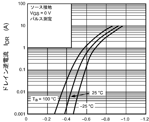
図 8.9 I_{DR} - V_{DS}
