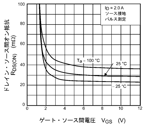
図 8.4 R_{DS(ON)} - V_{GS}
