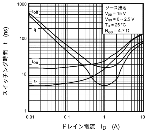
図 8.11 t - I_D
