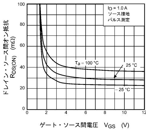
図 8.3 R_{DS(ON)} - V_{GS}
