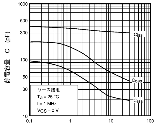
図 8.10 C - V_{DS}
