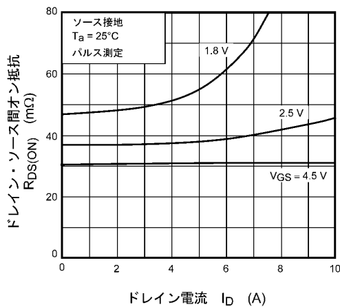
図 8.5 R_{DS(ON)} - I_D
