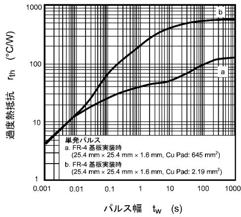
図 8.13 r_{th} - t_w
