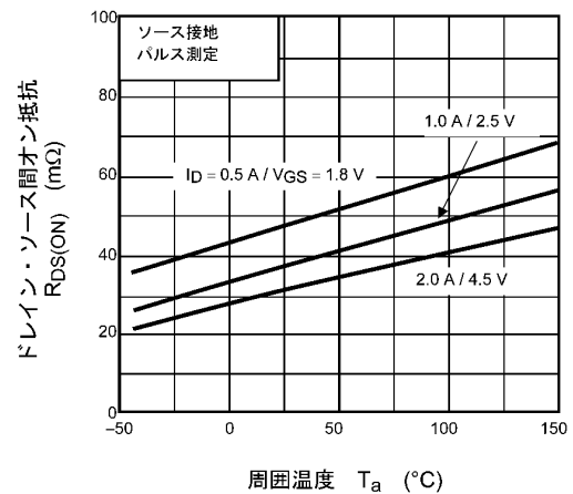
図 8.6 R_{DS(ON)} - T_a
