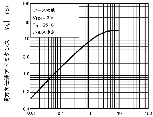
図 8.8 |Y_{fs}| - I_D
