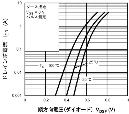
図 9.7 I_{DR} - V_{DSF}
