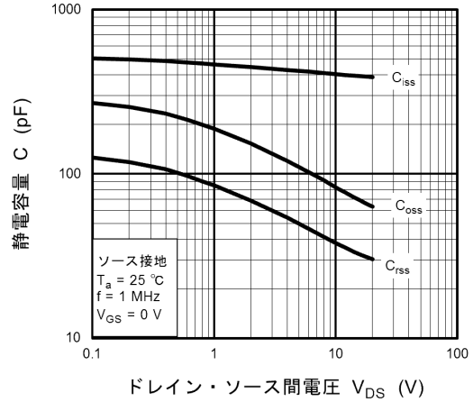
図 9.8 C - V_{DS}
