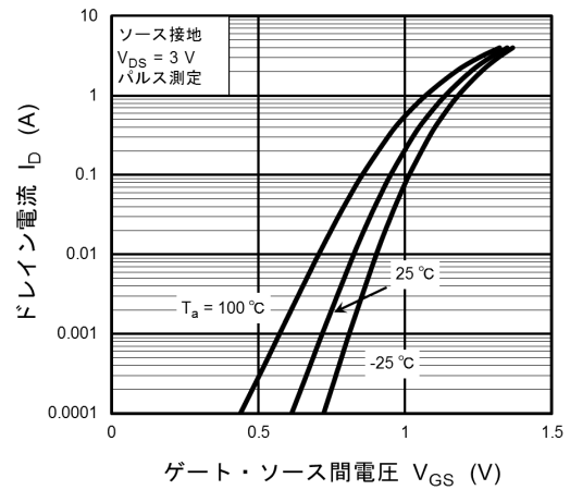
図 9.2 I_D - V_{GS}
