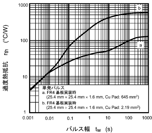
図 8.11 r_{th} - t_w
