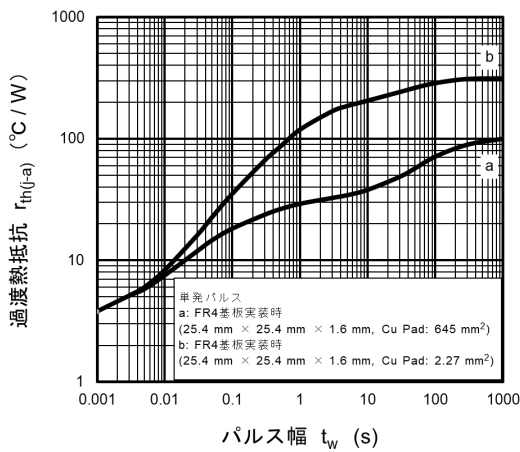
図 9.11 r_{th(j-a)} - t_w
