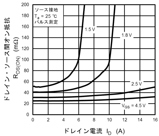
図 9.4 R_{DS(ON)} - I_D
