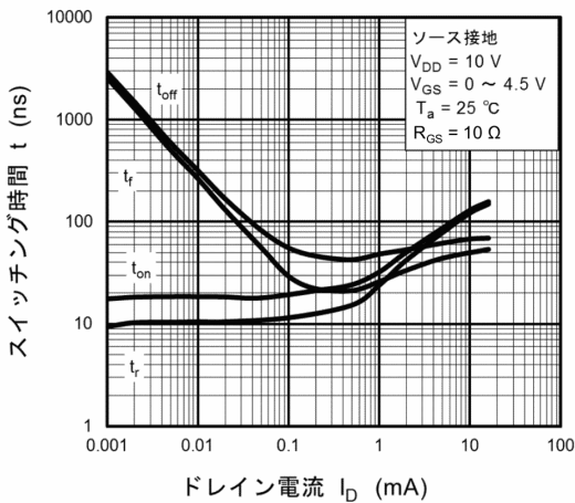
図 9.9 t - I_D
