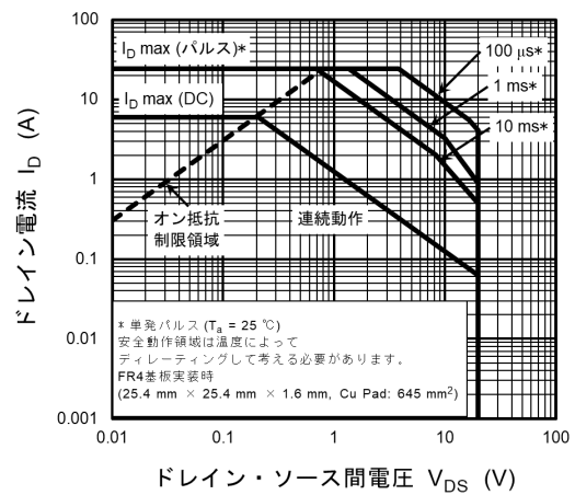
図 9.12 安全動作領域
