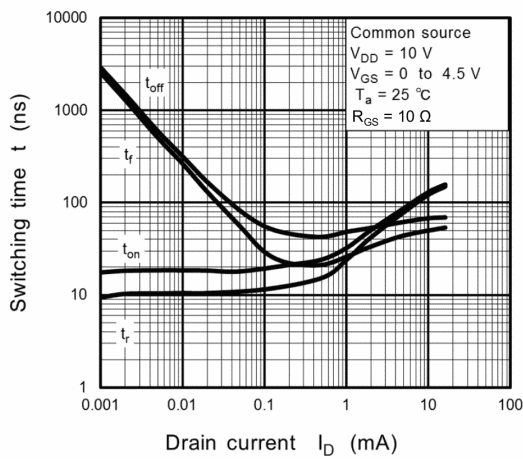
Fig. 9.9 t - I_D
