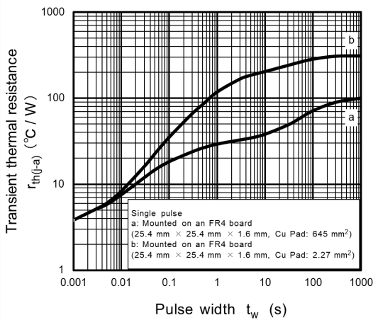
Fig. 9.11 r_{th(j-a)} - t_w
