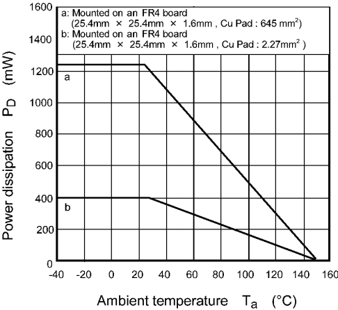
Fig. 9.13 P_D - T_a
