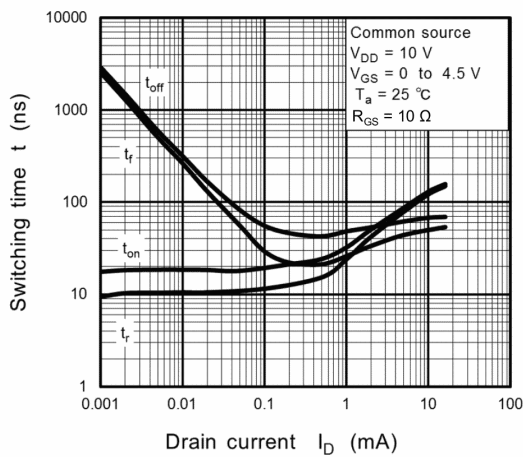
Fig. 8.9 t - I_D
