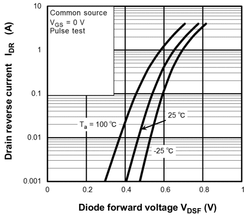
Fig. 9.7 I_{DR} - V_{DSF}
