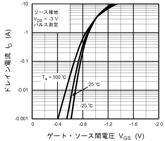
図 8.2 I_D - V_{GS}
