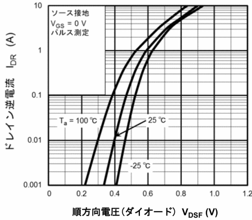
図 8.7 I_{DR} - V_{DSF}
