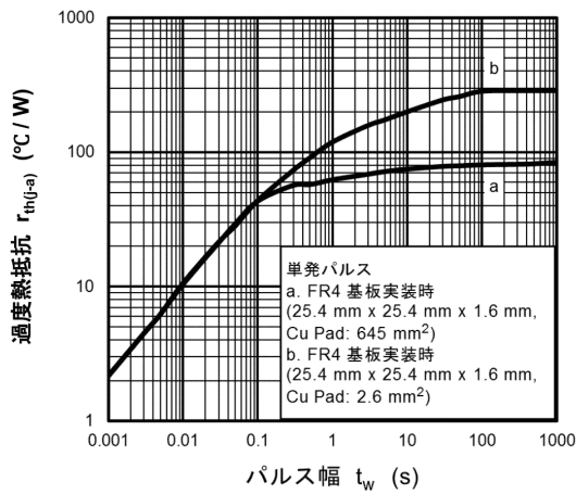
図 8.11 r_{th(j-a)} - t_w
