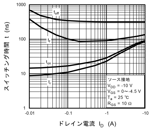
図 8.10 t - I_D
