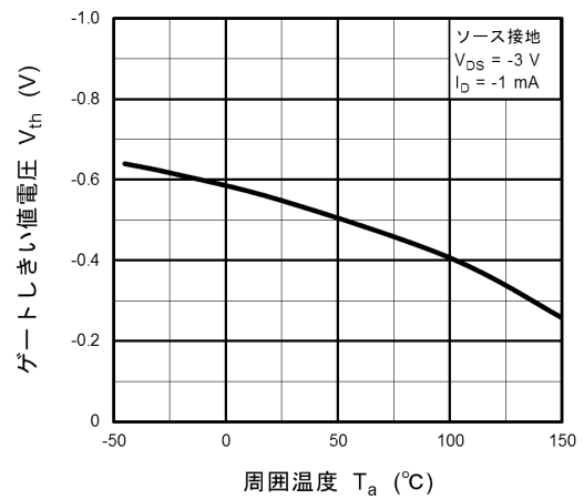
図 8.6 V_{th} - T_a
