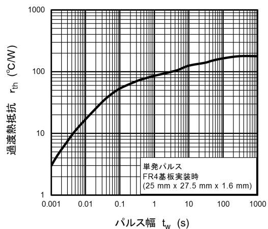
図 9.7 r_{th} - t_w
