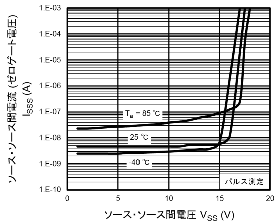
図 9.6 I_{CSS} - V_{SS}
