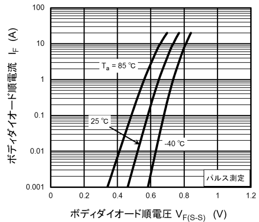
図 9.4 I_F - V_F
