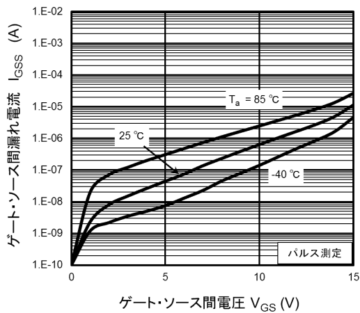
図 9.5 I_{GSS} - V_{GS}
