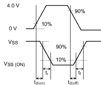
図 6.3.2 入力波形/出力波形
