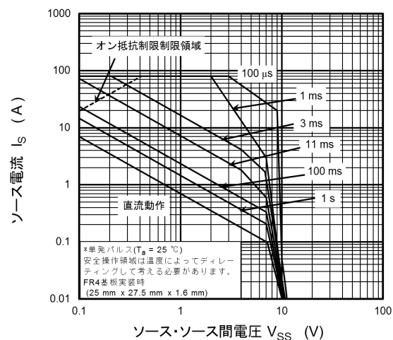
図 9.8 安全動作領域
