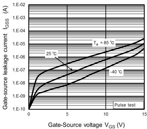
Fig. 9.5 I_{GSS} - V_{GS}
