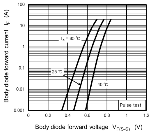
Fig. 9.4 I_F - V_{F(S-S)}
