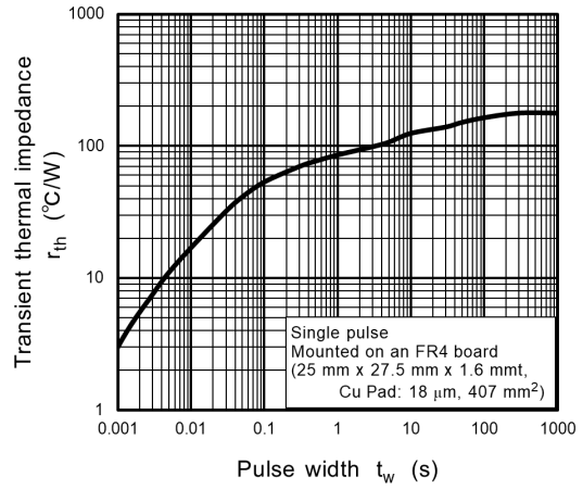
Fig. 9.8 r_{th} - t_w
