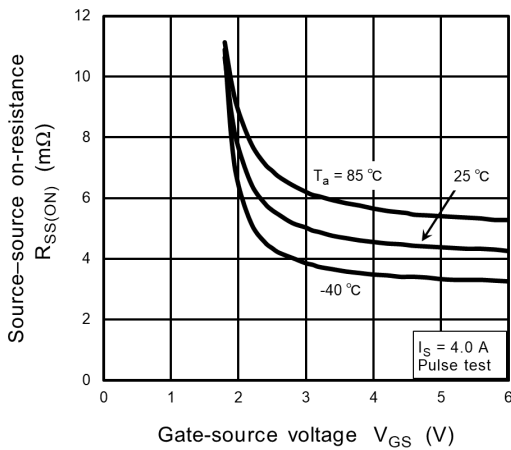
Fig. 9.3 R_{SS(ON)} - V_{GS}
