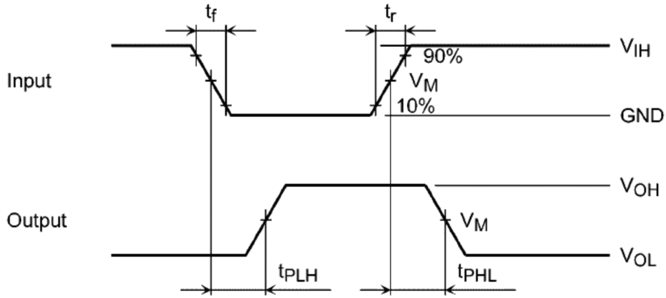
図 11.6.1 t_{PLH} , t_{PHL}
