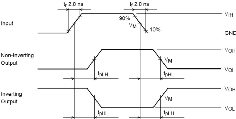
図 12.6.1 t_{pLH} , t_{pHL}
