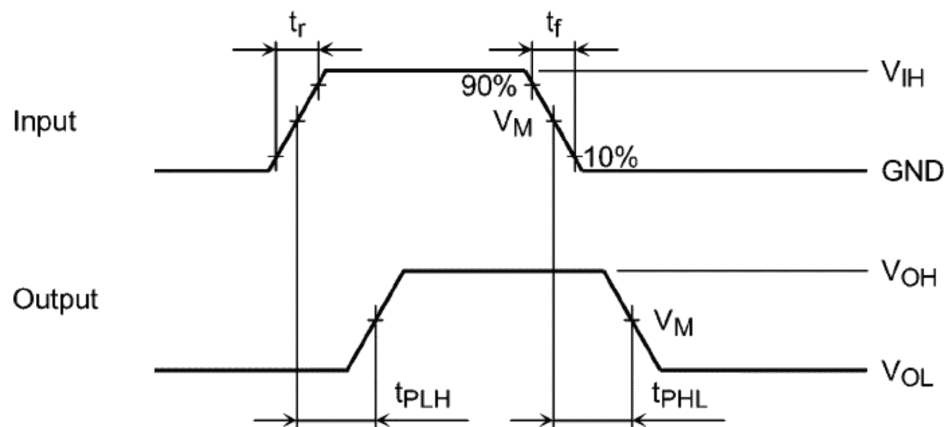
図 11.6.1 tPLH, tPHL
